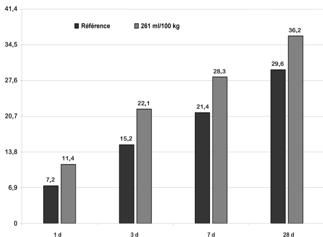
Résistance à la compression de PLASTOL 5700 (MPa)
