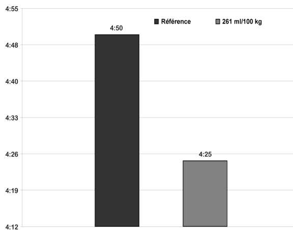
Temps de prise de PLASTOL 5700 (h:min)
